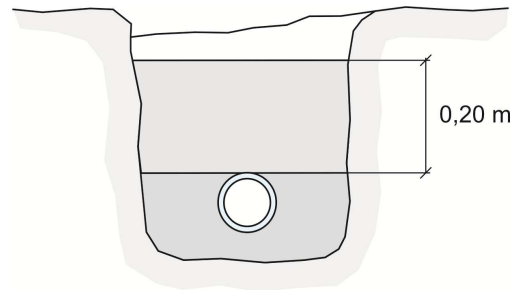
Fig. 8- Envolvimento da tubulação de polietileno PE
