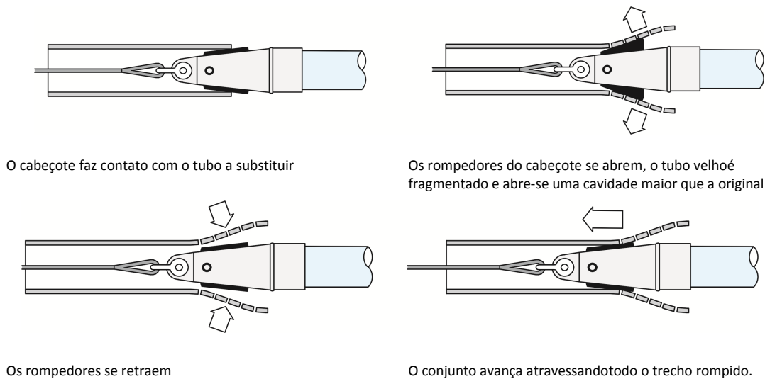
Fig. 6 -Esquema da técnica de pipebursting
