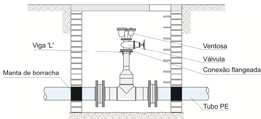
Fig.14 – Instalação de ventosas
