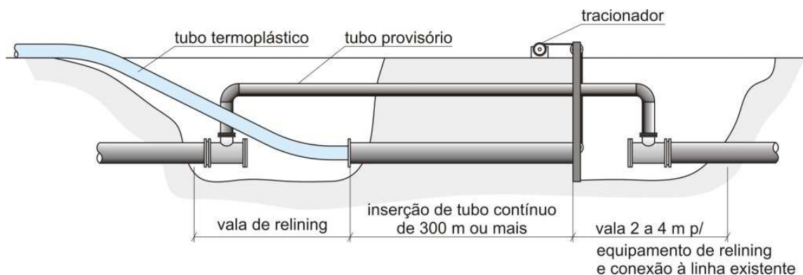
Fig. 4 - Esquema da típico da técnica de Relining ou sliplining
