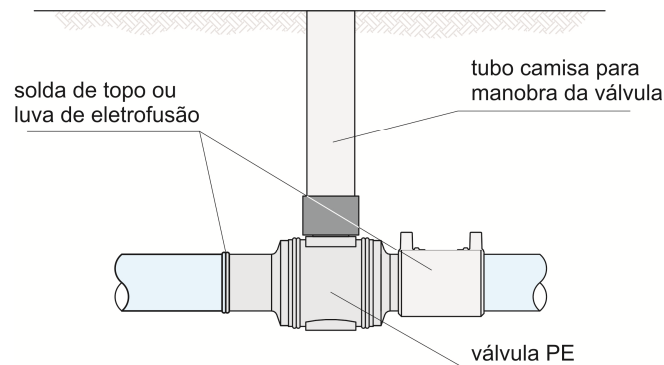
Fig. 13 – válvulas enterradas
