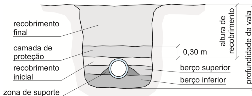
Fig.9- Envolvimento da tubulação de SDR> 17
