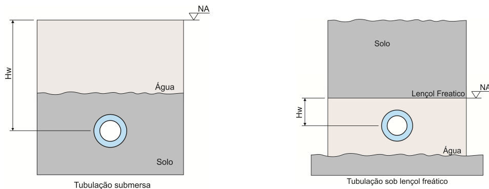
Fig. 8– Tubulação enterrada sob leito subaquático
