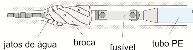
Fig.4 – Fusível mecânico para tração de tubulação
