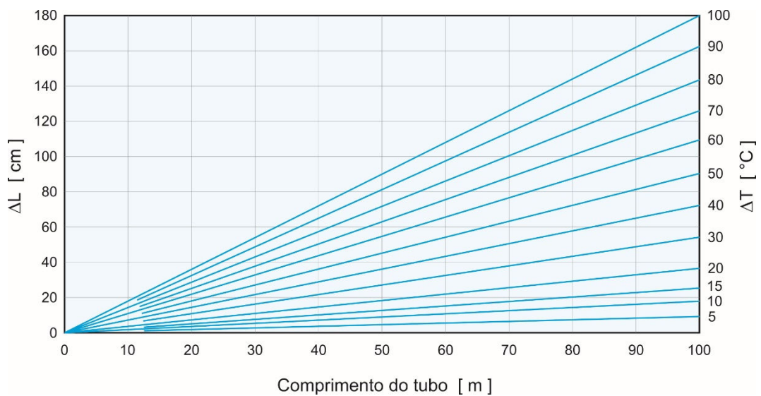
Fig.- Expansão térmica linear para tubos de PE e PP
