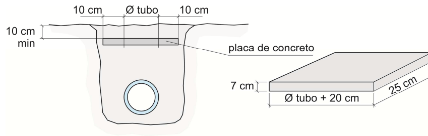
Fig.11- Placa de Concreto para proteção de tubulação
