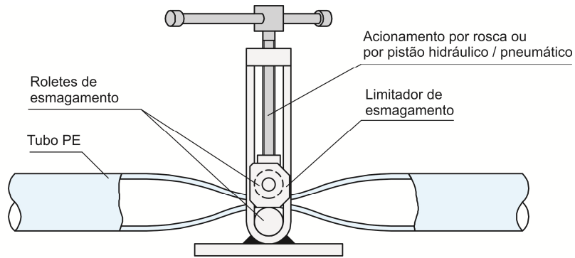
Fig.: Estrangulador de vazão
