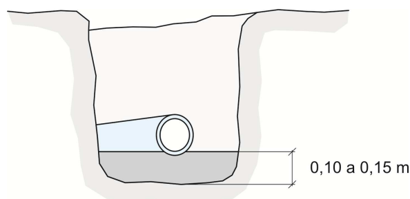
Fig.2 - Camada adicional de solo para cobrir fundo de vala
