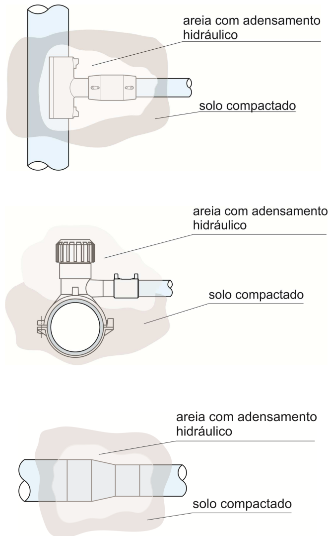
Fig.10- Assentamento e compactação de derivação
