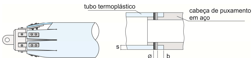
Fig 9– Cabeças de puxamento
