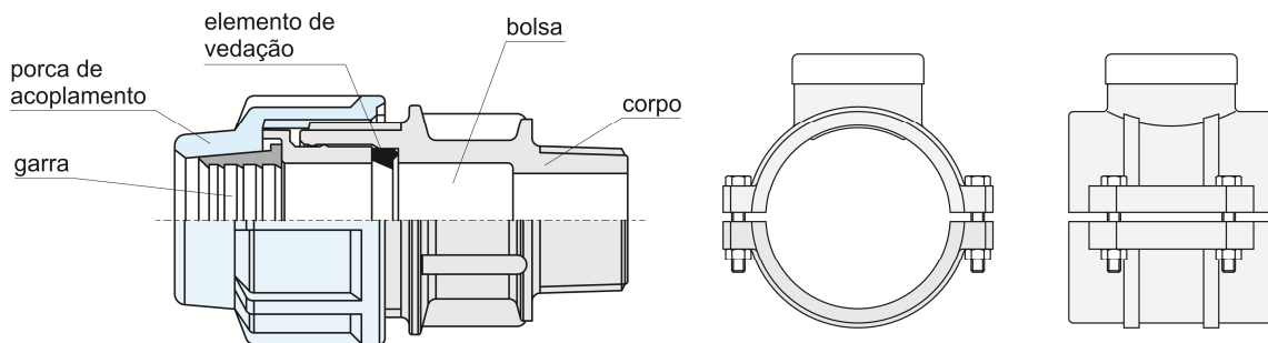
Conexão de Compressão
