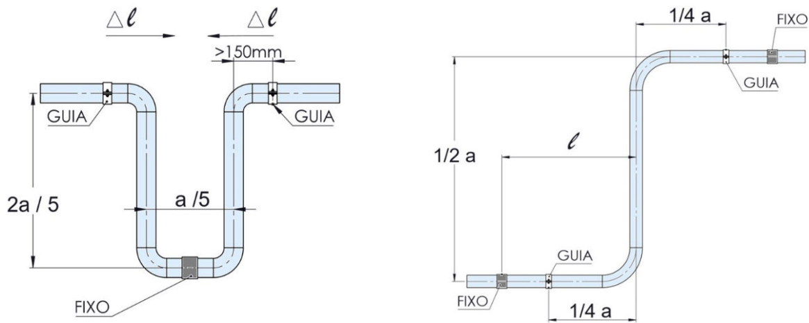
Fig.- Instalação com Efeito Lira.
