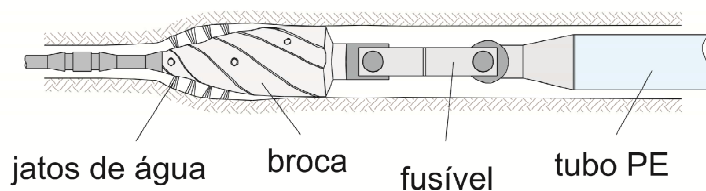
Fig. 2 - Sonda de perfuração
