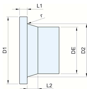
Colarinho (Adaptador de Flange)
