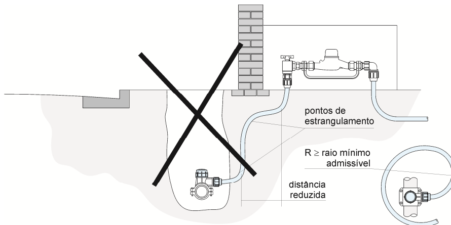
Fig.17 - Assentamento do tubo em distâncias reduzidas
