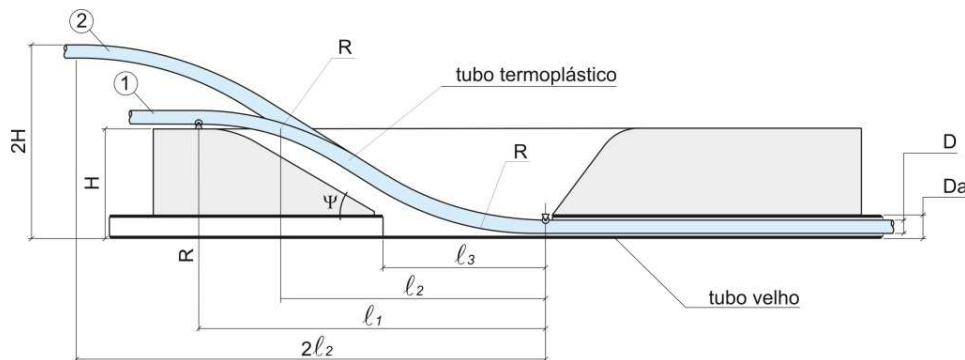
Fig.7 -Esquema e dimensionamento de vala para Inserção
