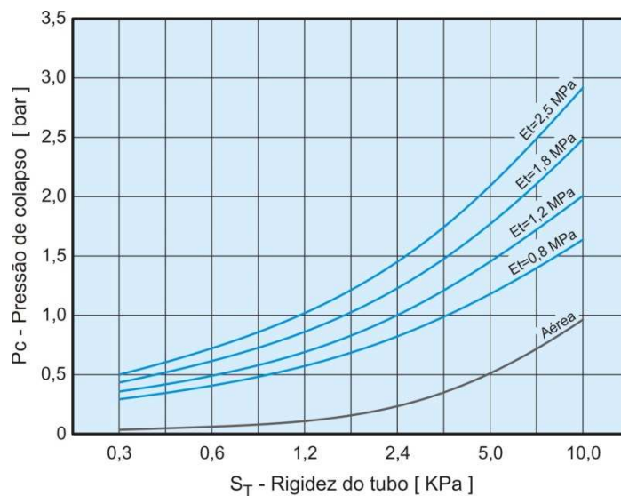
Fig. 8– Gráfico de P_C em função da Rigidez do tubo ( S_T )
