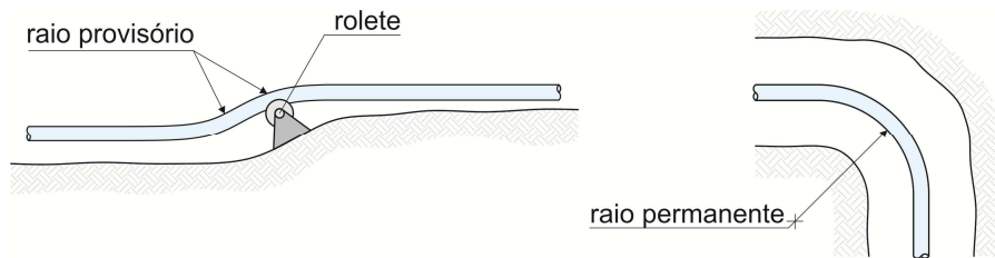
Fig.7– raio de curvatura de tubos
