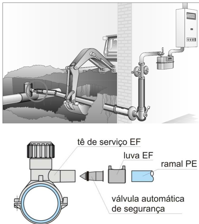
Fig.18 – Válvula Automática de Segurança
