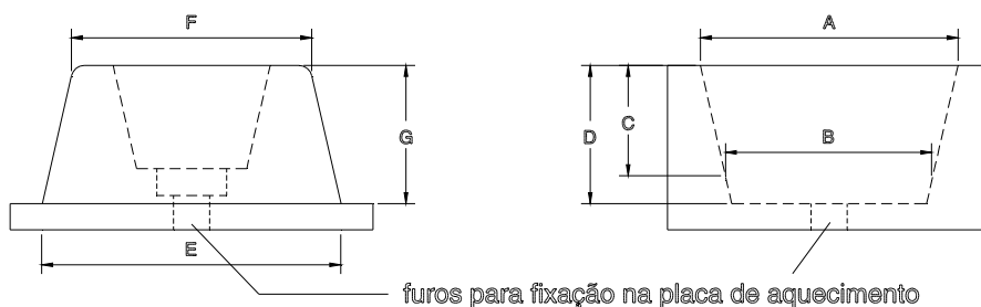
Dimensões dos gabaritos de aquecimento para solda soquete
