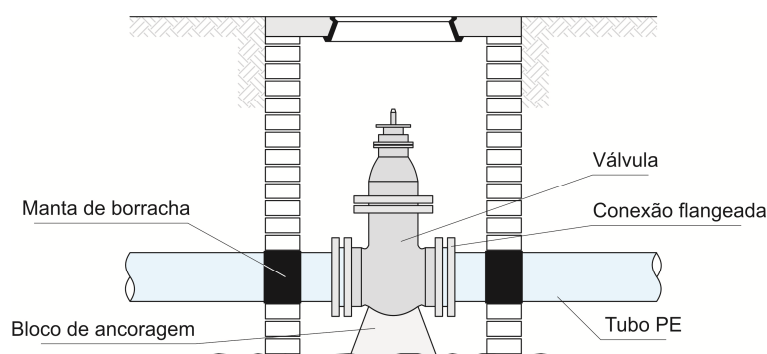
Fig.12- Ligações de válvulas em caixas
