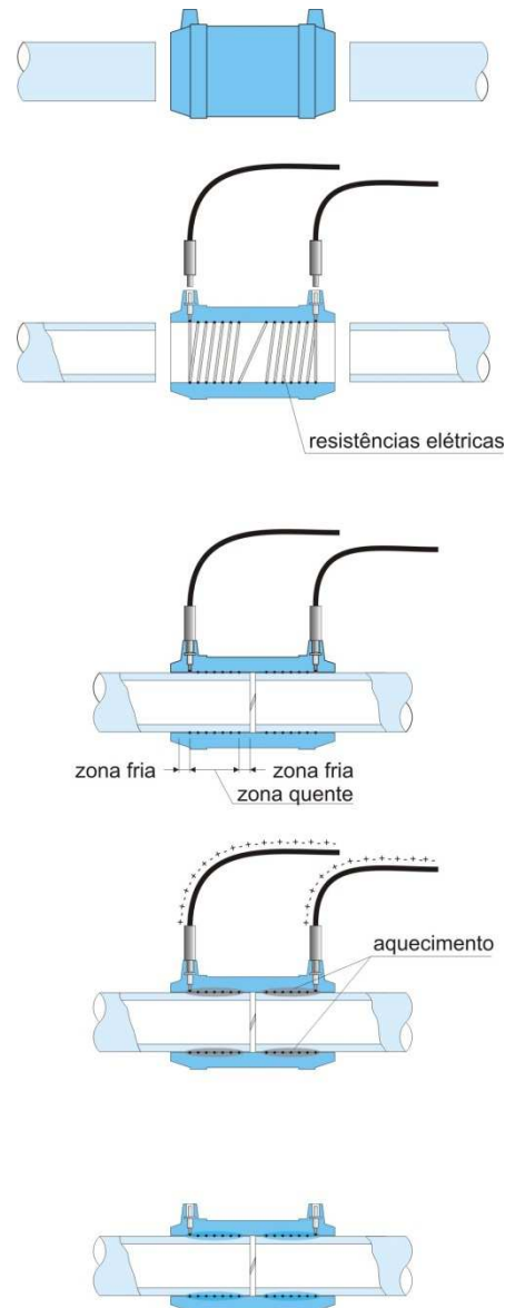
O Princípio da Soldagem por eletro fusão
