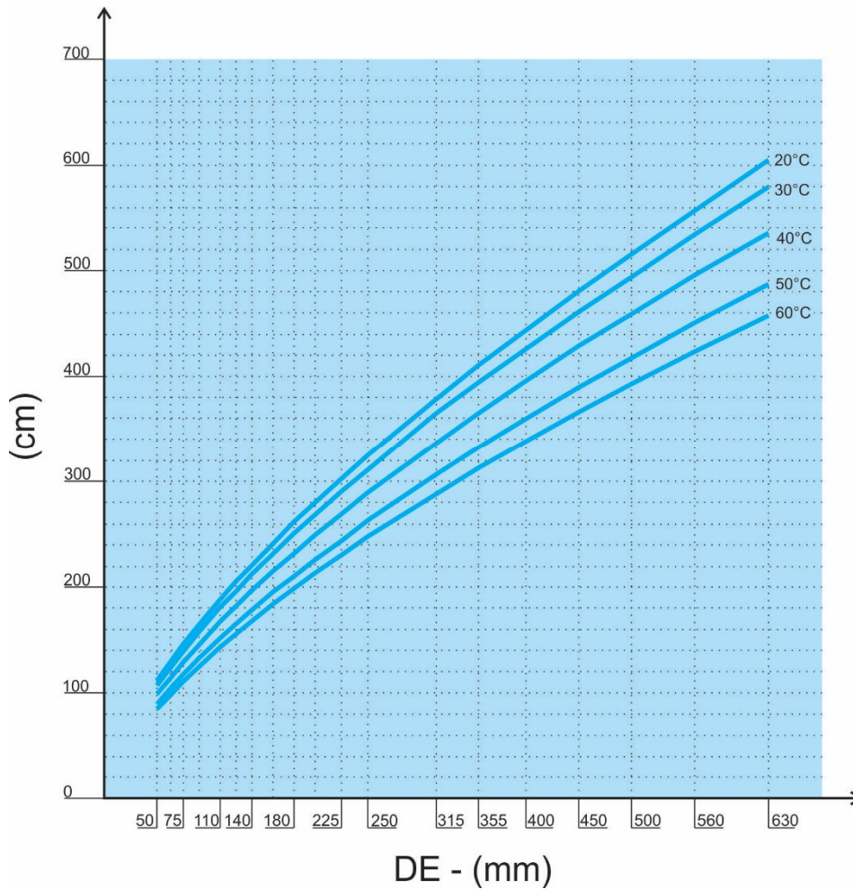
Fig. – Distância entre apoios para tubos cheios de água
