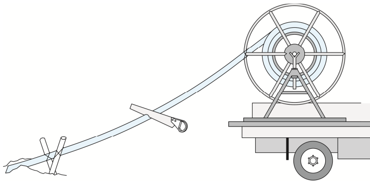
Fig.3– carretel para aplicação de tubos em bobinas
