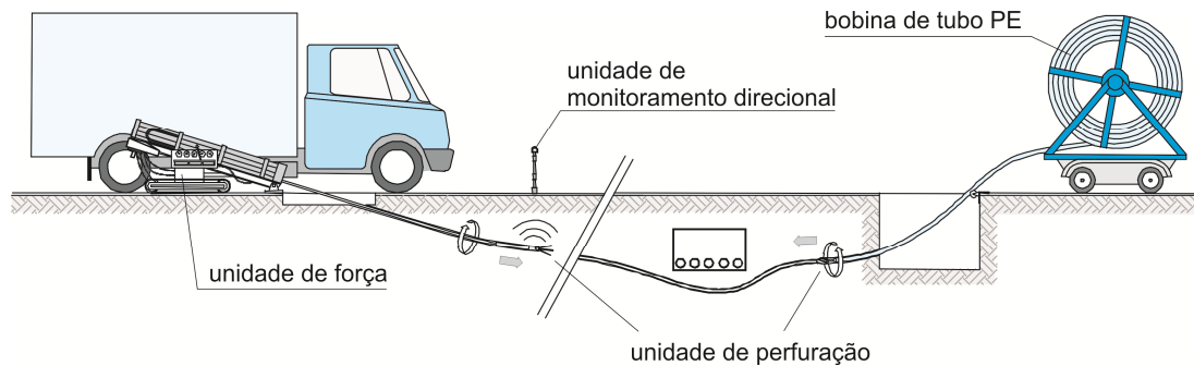
Fig. 1 - Esquema da Operação de Furo Direcional
