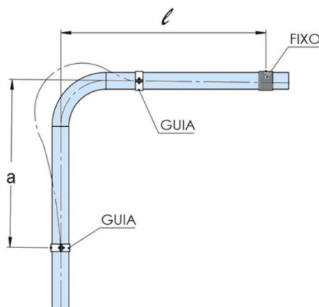
Fig– Dilatação em Tês e curvas
